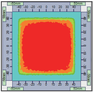
橫切面照度分佈
