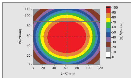
▲ HCNS-200-W
